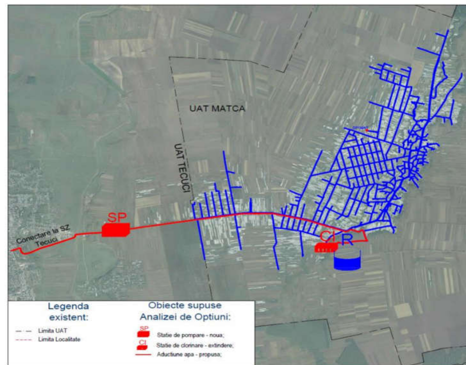
Optiunea 2 - Alimentare cu apa localitatea Matca.
